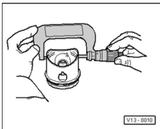
Fig. 140: Checking Piston
