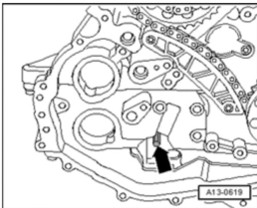
Fig. 171: Press Tube 30 - 100
