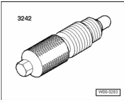
Fig. 165: Crankshaft Holder 3242
