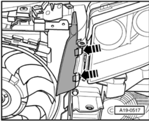
Fig. 440: Air Guides
