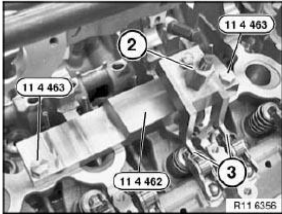
Fig. 259: Pressing Rocker Arms
